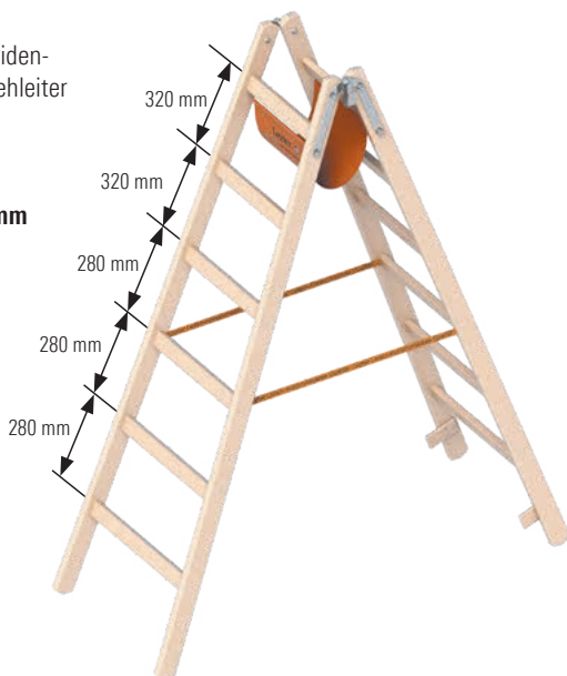
Holzstehleiter 1053 nach Ö-Norm Z1501
